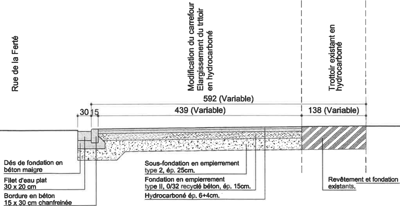
Coupe type A-A projetée. Ech. 1/50
